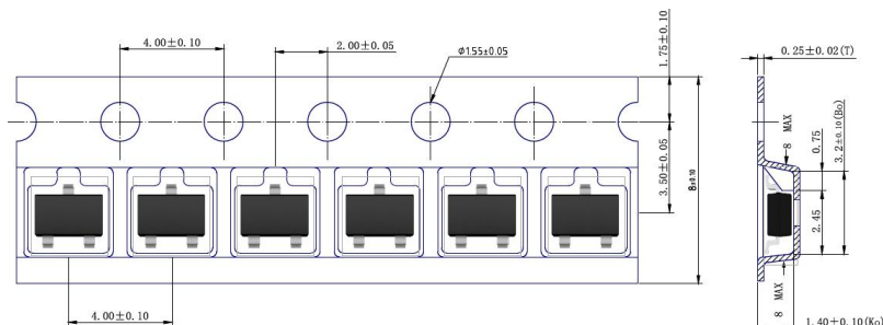
Reel (7")
