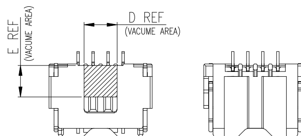
2PIN~5PIN
