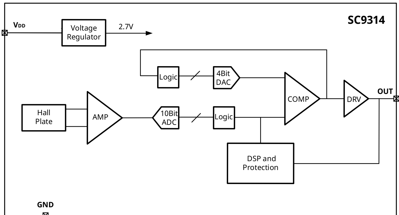
图 3 功能框图
