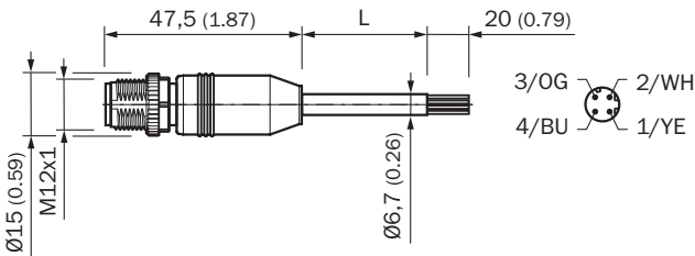
尺寸图 (尺寸单位: mm)
