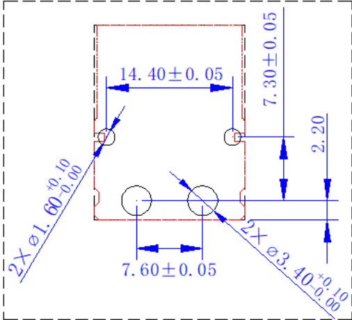
互配尺寸
