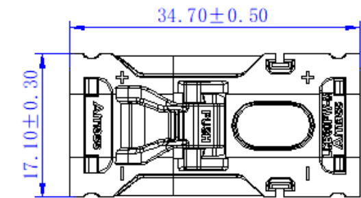
互配尺寸
