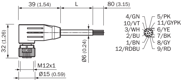
尺寸图 (尺寸单位: mm)
