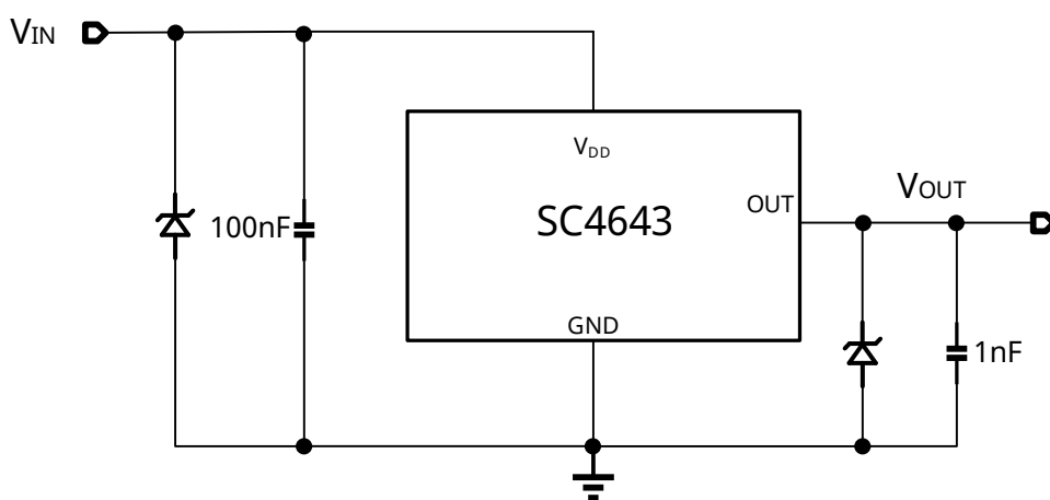
图 7. TO92U 典型应用线路图
