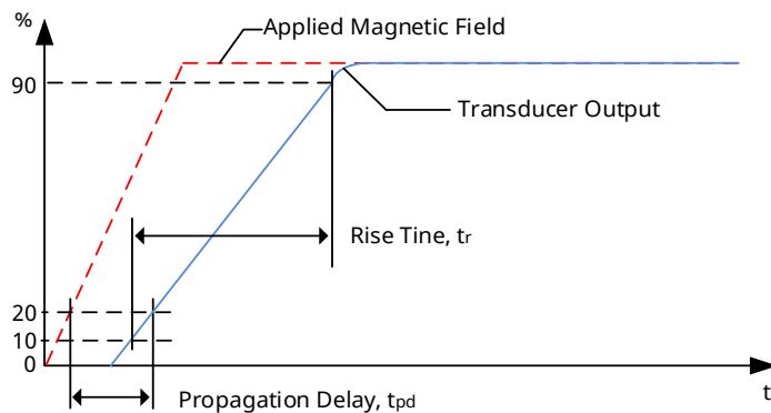
图 5. 传播延迟和上升时间定义
