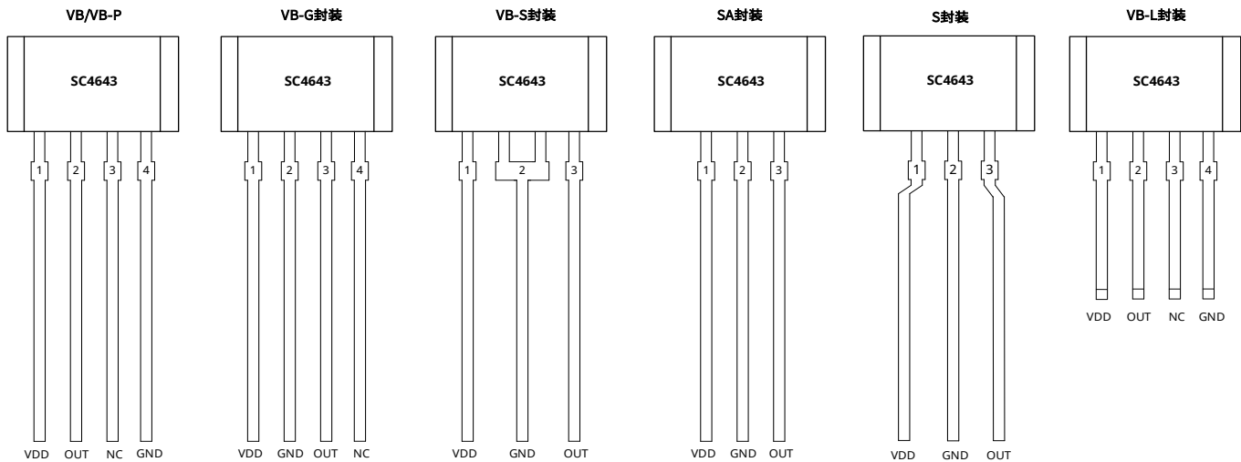
图 2. 封装俯视图
