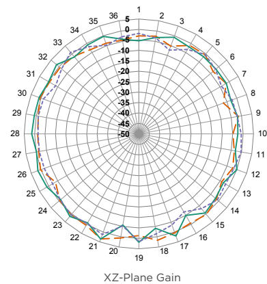
XZ-Plane Gain
