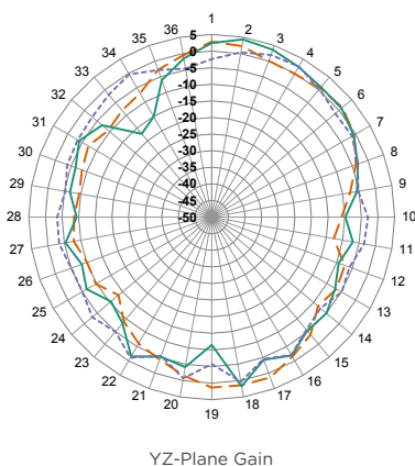
YZ-Plane Gain
