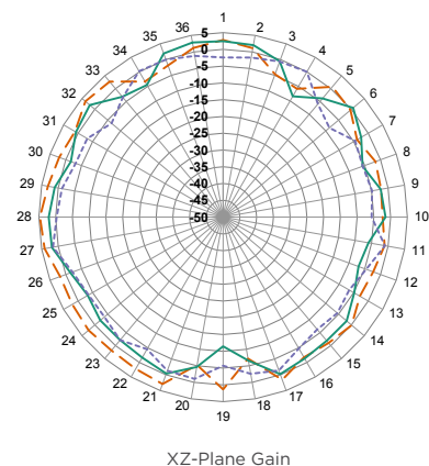
XZ-Plane Gain
