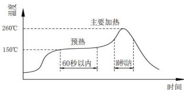
图 8. 回流炉温度设置条件
