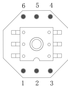
图 1. 引脚示意图(俯视图)
