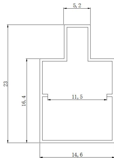
图 9.料管截面示意图
