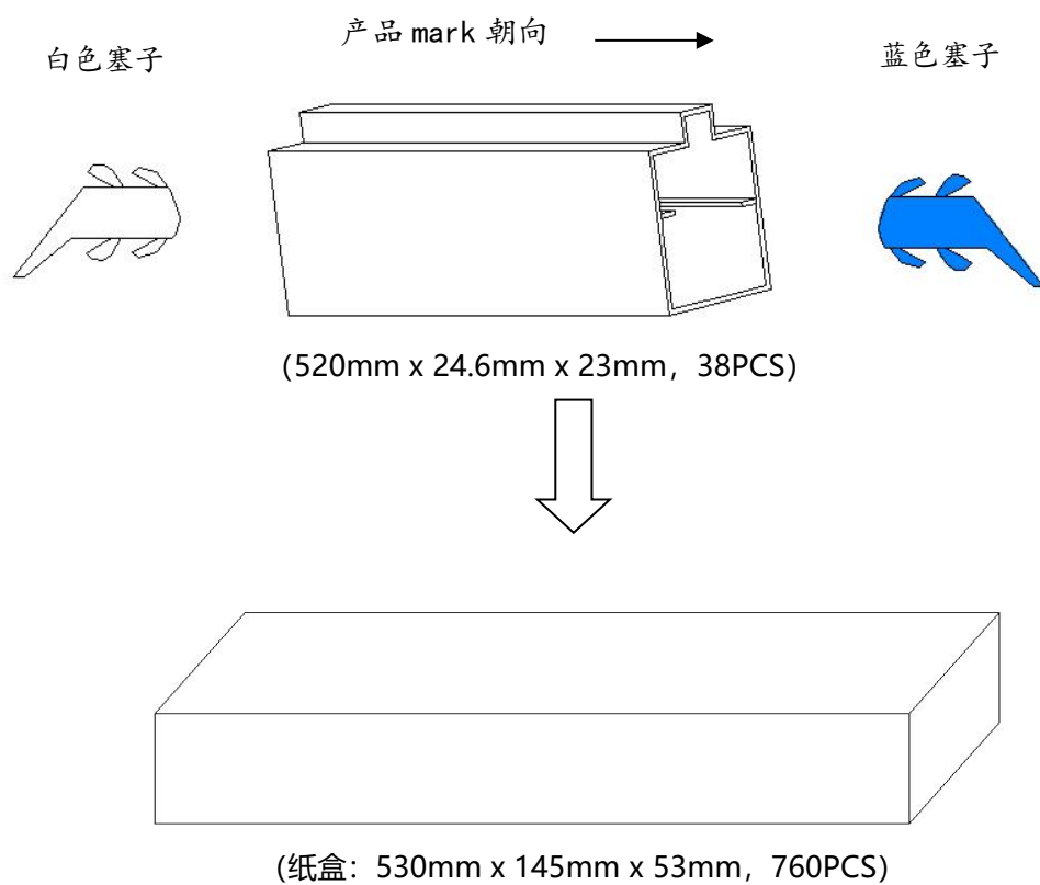
图 10.包装示意图
