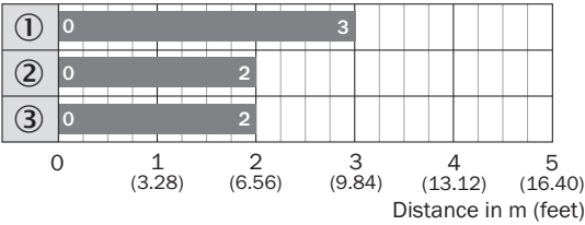
触发感应距离图表 (MDO 5 mm)
