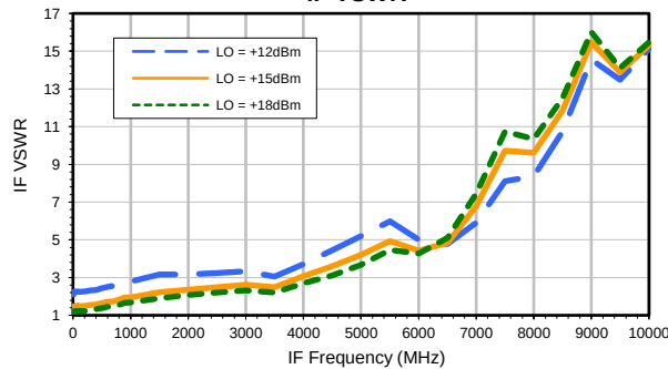
IF VSWR
