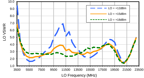
LO VSWR
