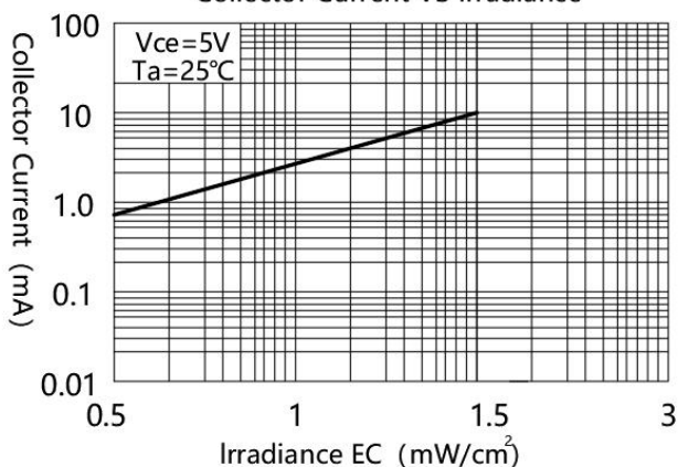
集电极电流与辐射强度的关系 Collector Current VS Irradiance
