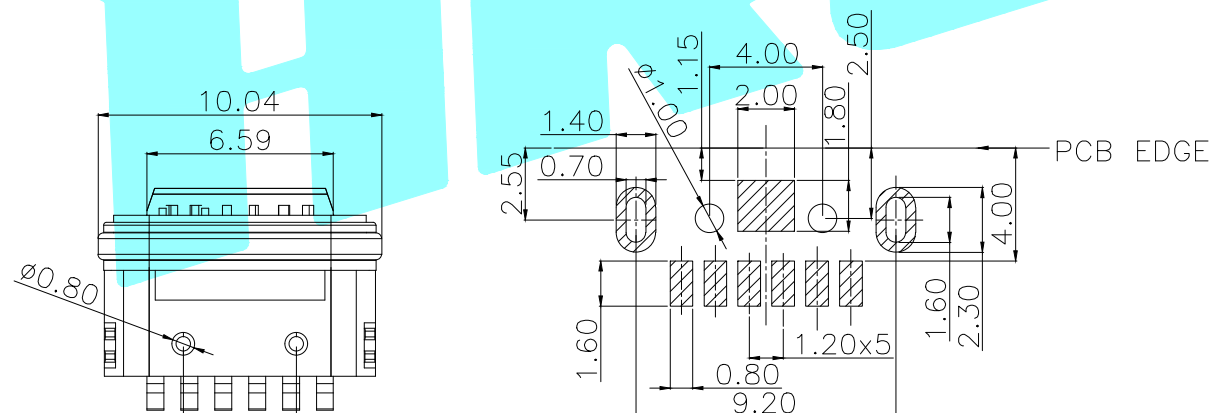
PCB Layout(Pattern side)
