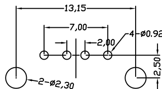
P.C.B Layout
