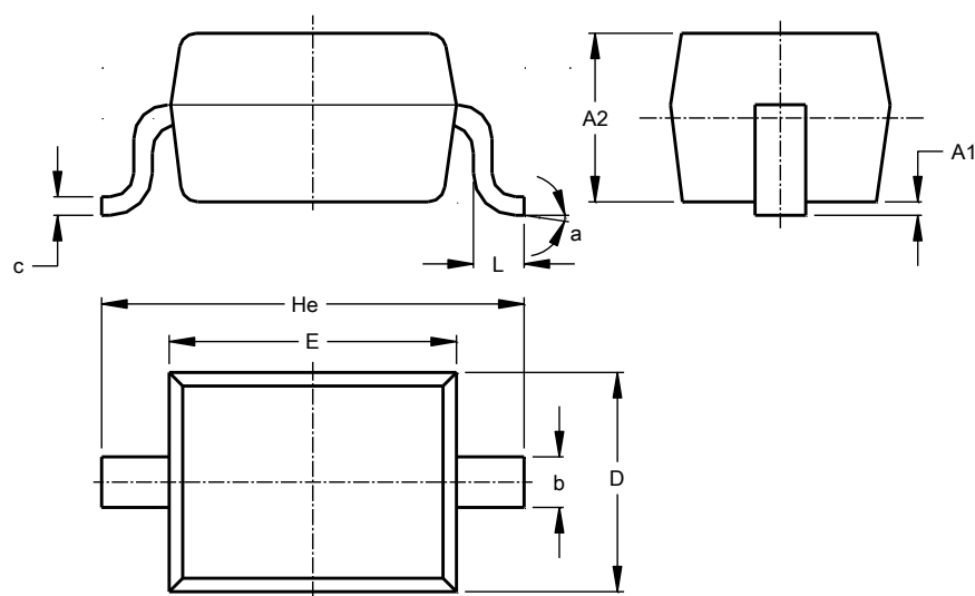
SOD323
