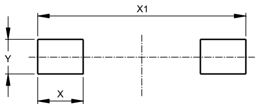
SOD323
