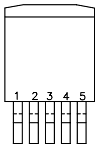
TO-263-5
