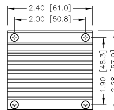
HAE75-□□S□□W - HS5 7GA0128P01-F
