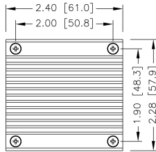
HAE75-□□S□□W - HS 7G-0021A-F
