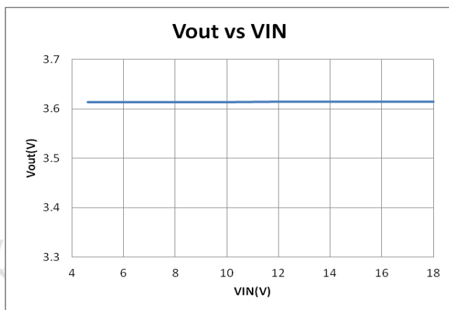
图9. 输出电压 与 输入电压
