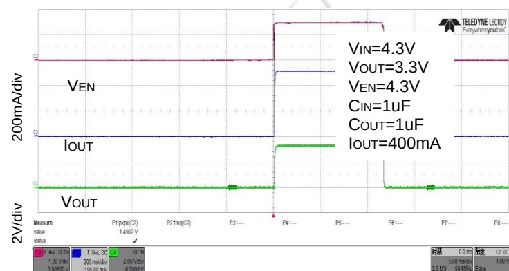
图 13. 使能开启响应
