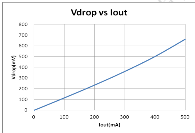
图 10. 压差 与 输出电流
