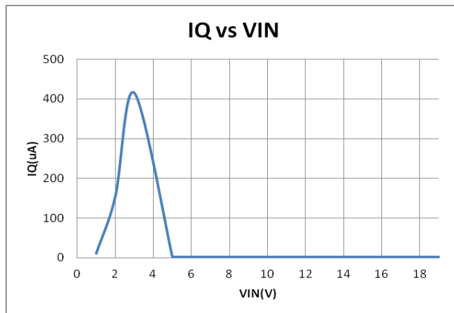
图 11. 静态电流 与 输入电压
