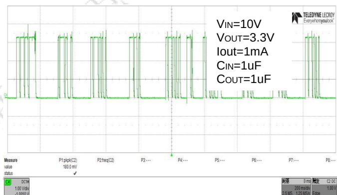
图 18. 连续热插拔输出过冲
