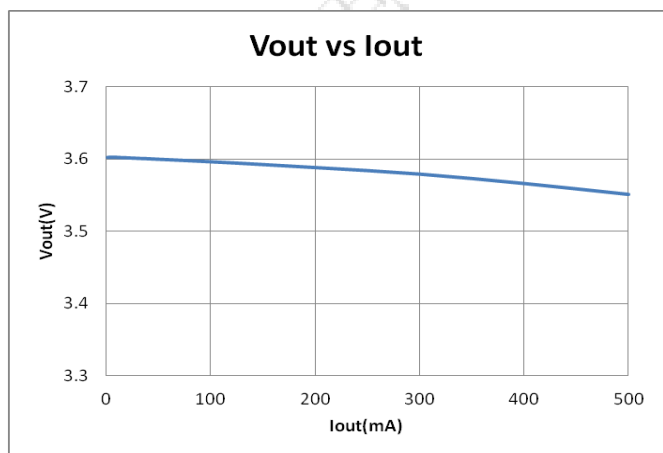
图8. 输出电压 与 输出电流
