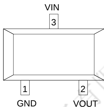
SOT23-3
