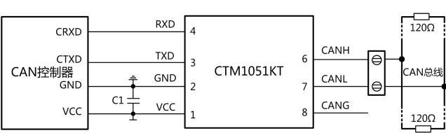
图 1. CAN 控制器 5V 供电应用电路
