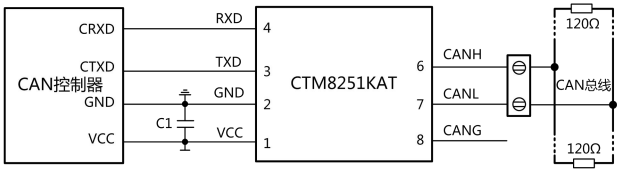
图 2. CAN 控制器 3.3V 供电应用电路
