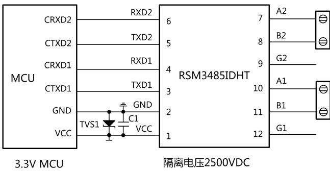
图 2.MCU 3.3V 供电应用电路
