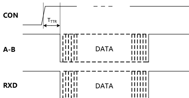
图 2. RSM(3)485CT模块数据接收时序图
