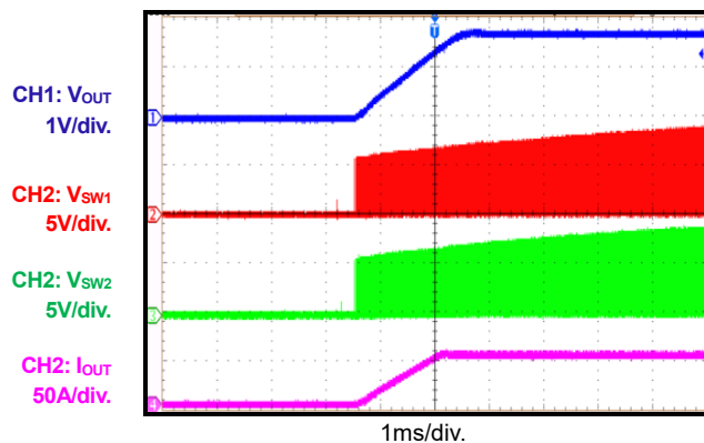
VIN Start Up, I_o=50A
