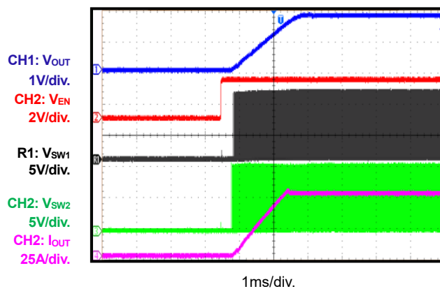
EN Start Up, I_o=50A
