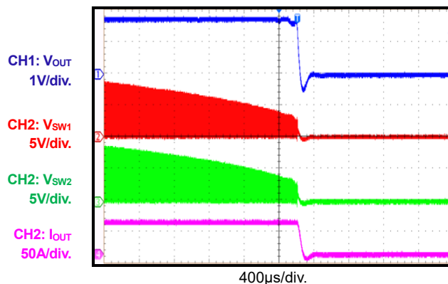
VIN Shutdown, I_o=50A
