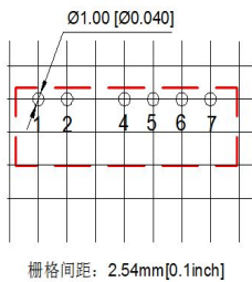
推荐 PCB 图
