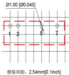
推荐 PCB 图
