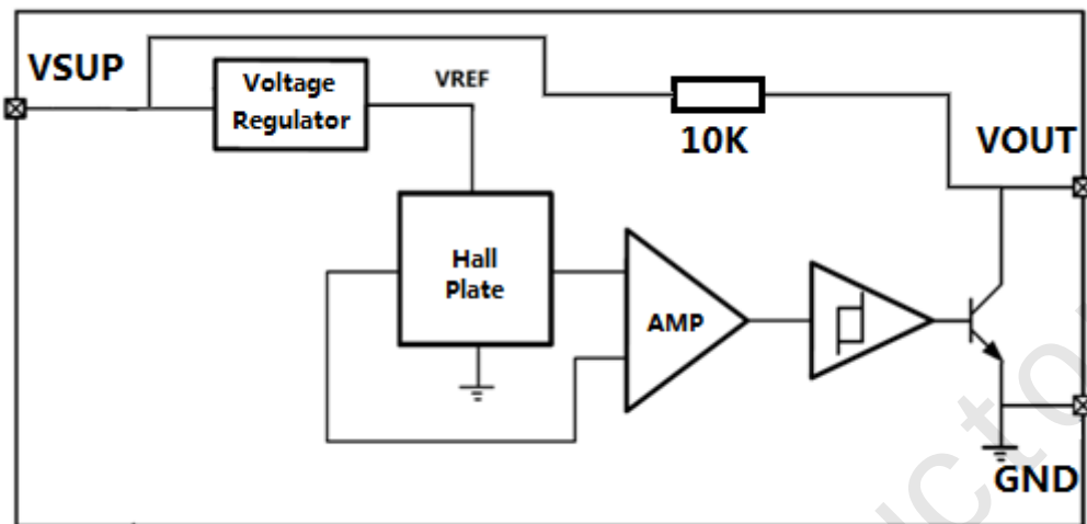
SS360PT功能框图
