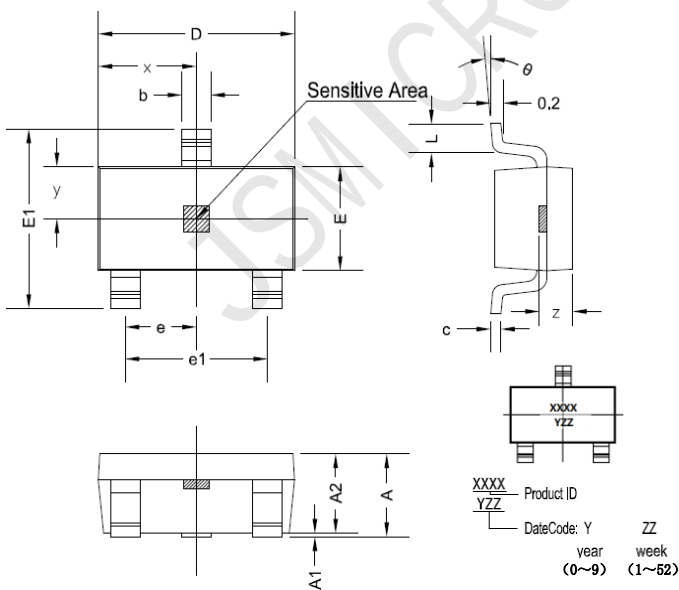
SOT23封装尺寸
