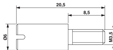
尺寸图
