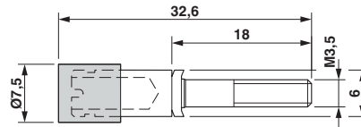
尺寸图
