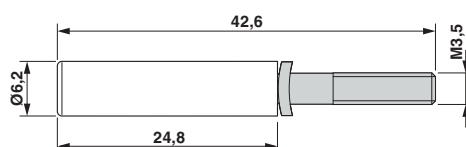
尺寸图
