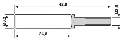
尺寸图
