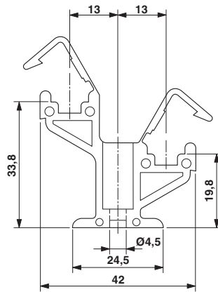
尺寸图
