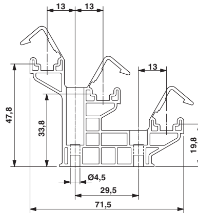
尺寸图
