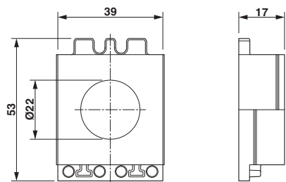
尺寸图
