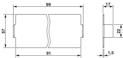
尺寸图
