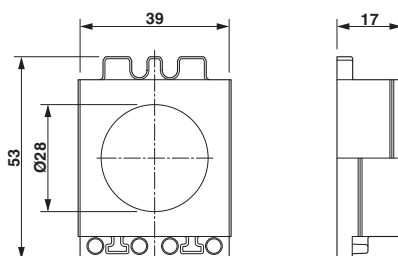
尺寸图
