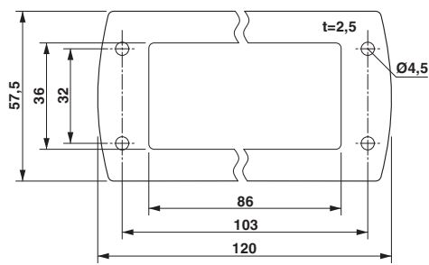
尺寸图
