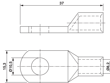
尺寸图
