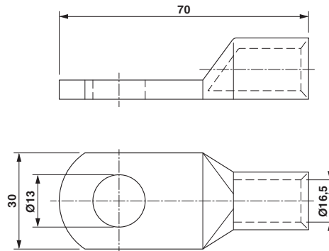
尺寸图
