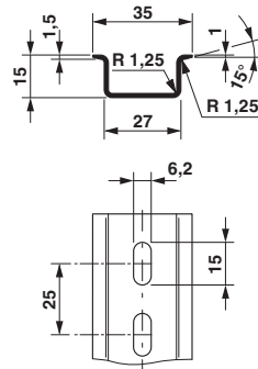
尺寸图
