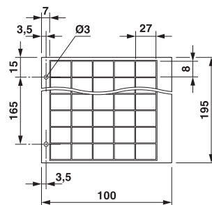
尺寸图
