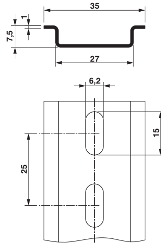
尺寸图
