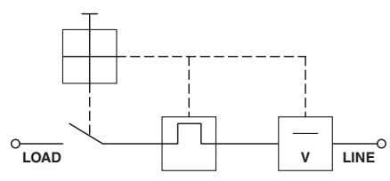
结构框图
