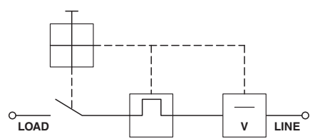
结构框图
