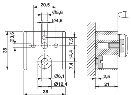
尺寸图
