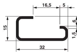
尺寸图
