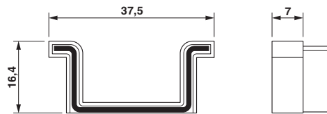
尺寸图
