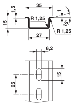
尺寸图
