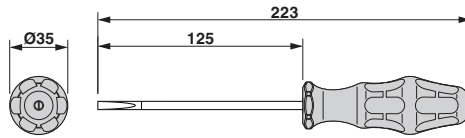
尺寸图
