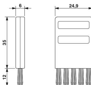
尺寸图
